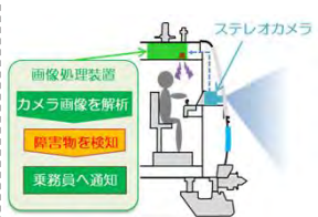
車両搭載型障害物検知システム
