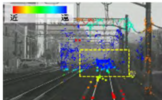
車両搭載型障害物検知システム
