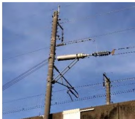
新幹線電車線（架線）設備
