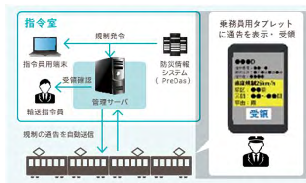
運転規制通告伝達システム
